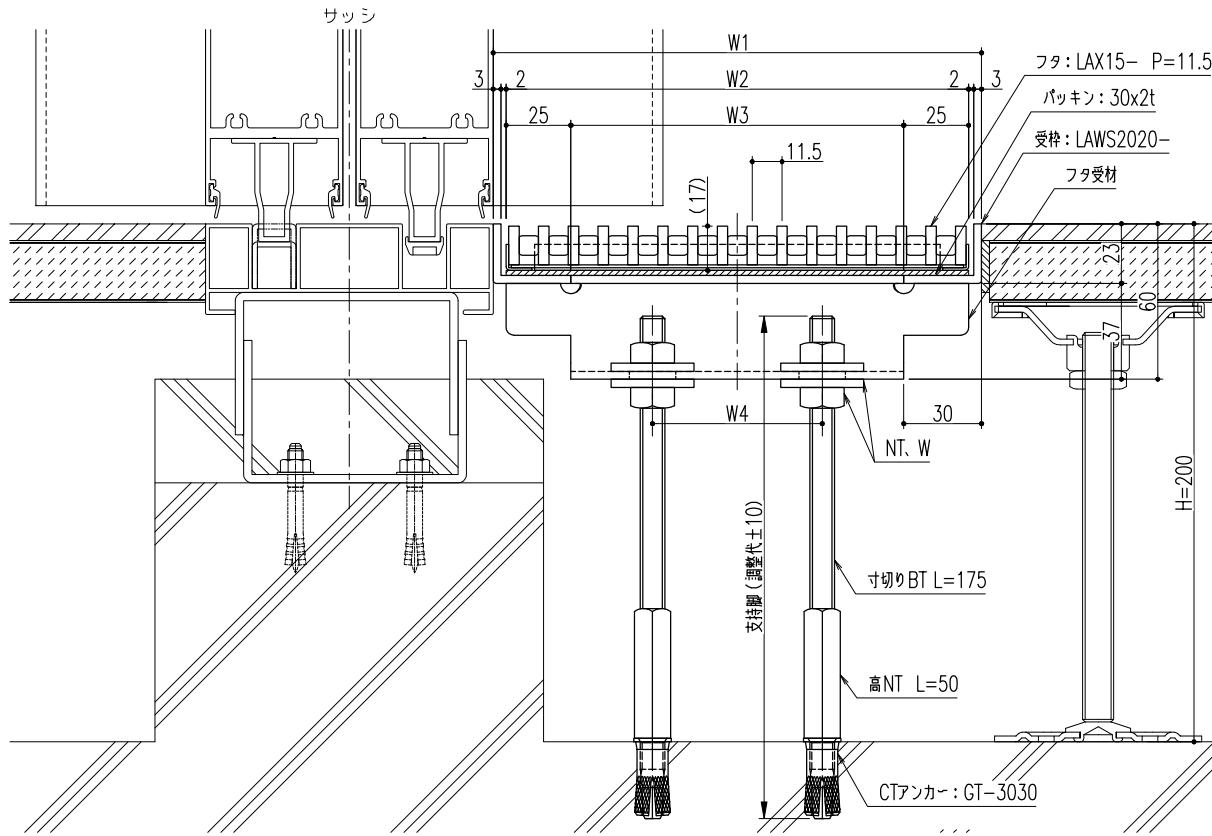
断面詳細図 (参考納まり図) S=1/2
