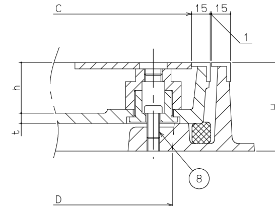
取手部断面拡大図
