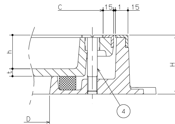
ボルト固定部詳細
