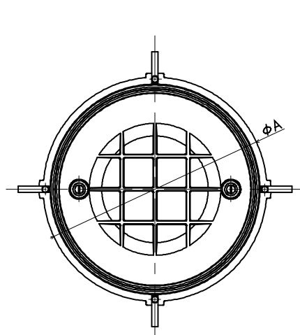
平面図（呼称450）
