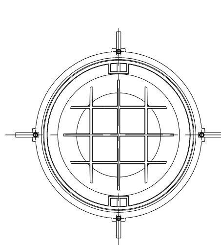
平面図(呼称450)
