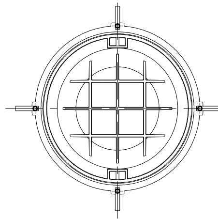
平面図(呼称450)
