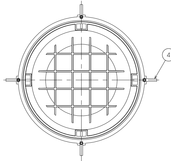
平面図(呼称600)
