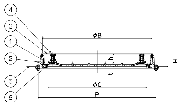
平面图(呼称600)
