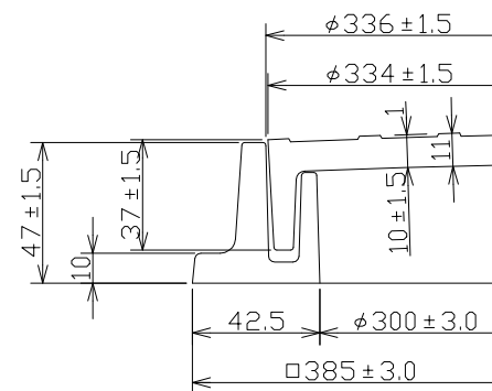
蓋・受枠断面詳細図
