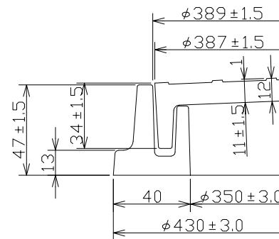
蓋・受枠断面詳細図
