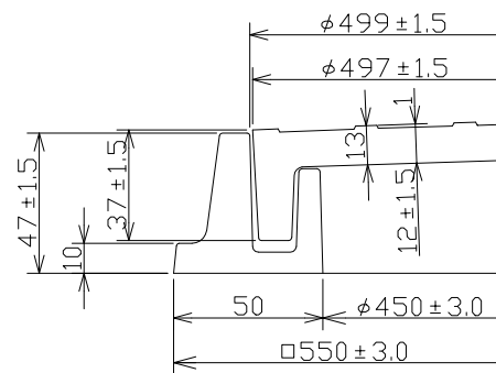
蓋・受枠断面詳細図
