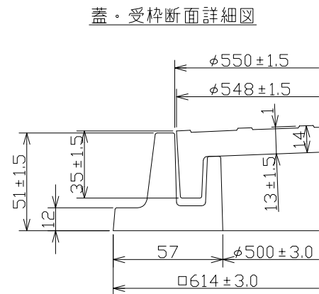
蓋・受枠断面詳細図
