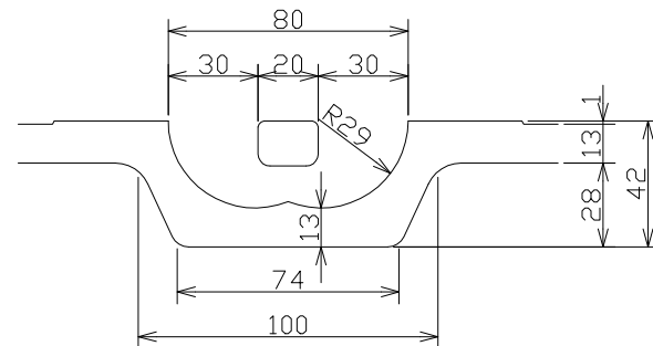
蓋・受枠断面詳細図
