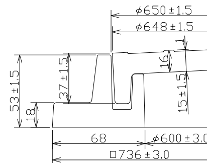
蓋・受枠断面詳細図
