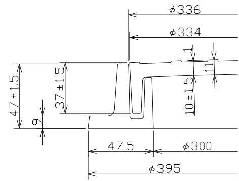
蓋・受枠断面詳細図
