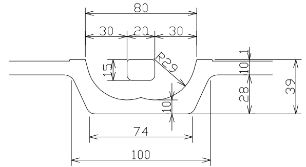
取手断面詳細図
