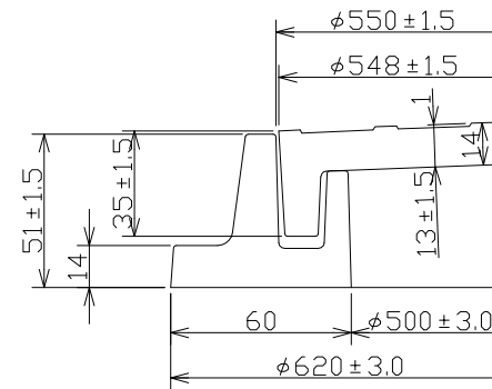
取手部断面詳細図
