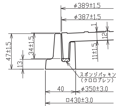
取手部断面詳細図
