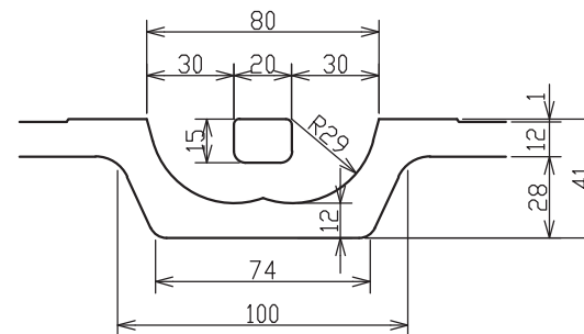
取手部断面詳細図
