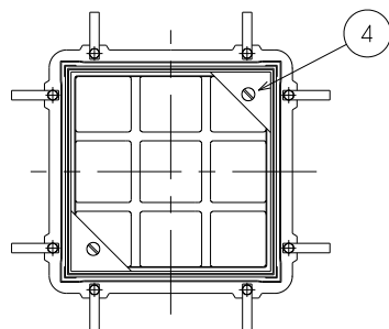
サイズ350/450平面図
