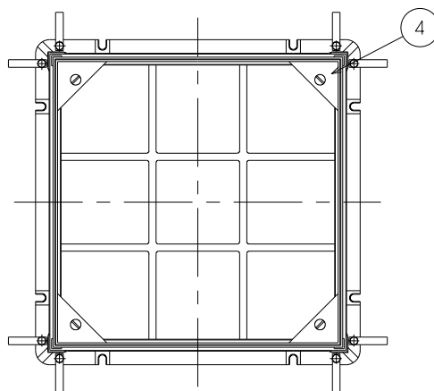
サイズ600平面図
