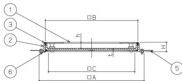
断面図
