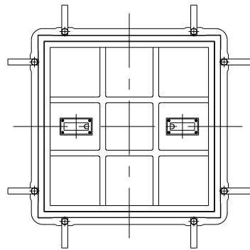
呼称450平面図
