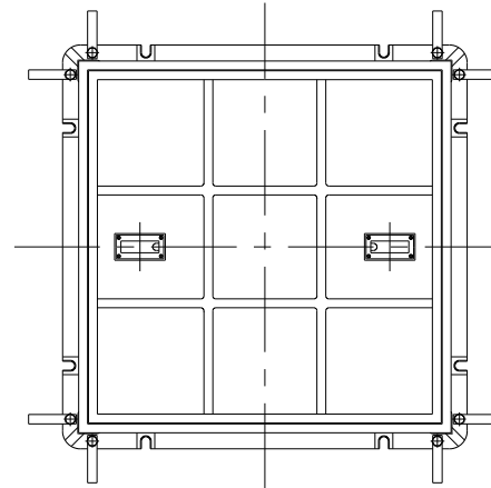
呼称600平面図
