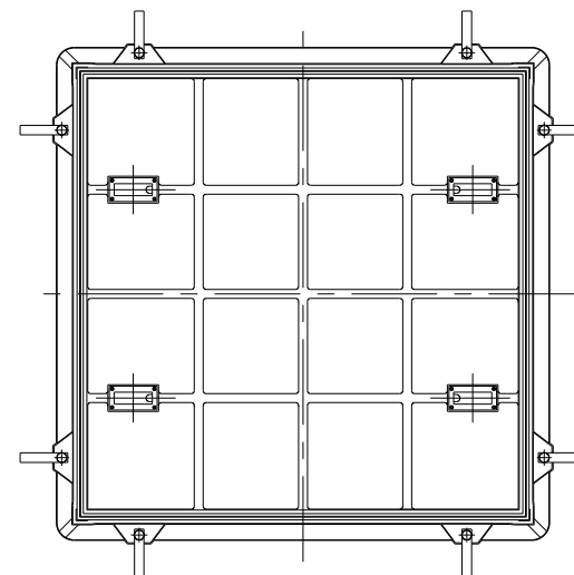
サイズ750平面図
