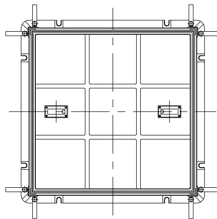
サイズ600平面図
