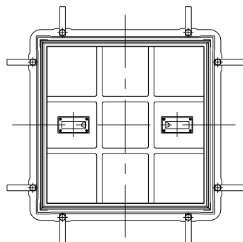
サイズ450平面図
