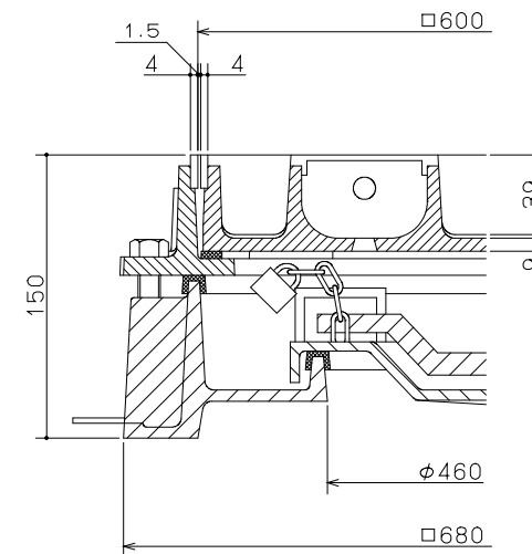
断面拡大図
