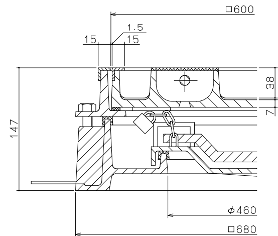
断面拡大図
