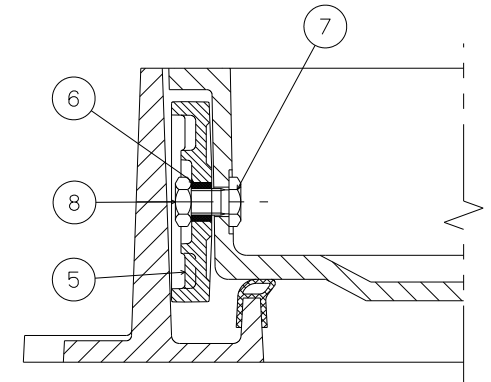
断面Z-Z
