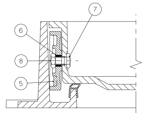
断面Z-Z
