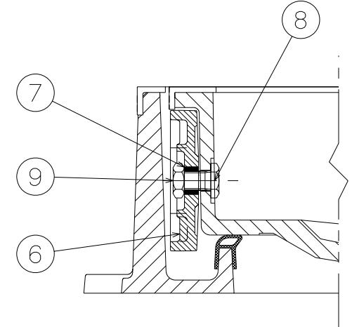
断面Z-Z
