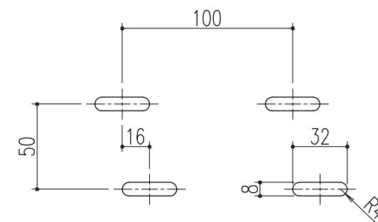
排水穴形状
