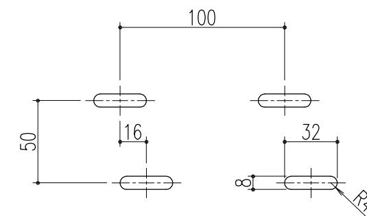
排水穴形状
