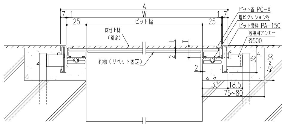
断面詳細図 S=1/2
