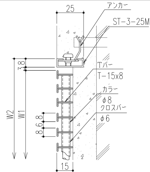
断面詳細図 S=1/2
