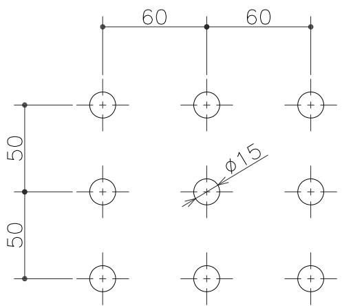
排水穴形状
