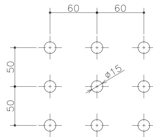
排水穴形状
