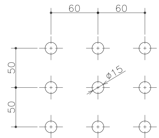
排水穴形状
