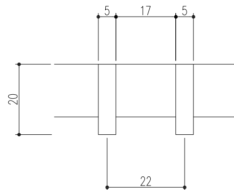
ベアリングバー断面詳細図
