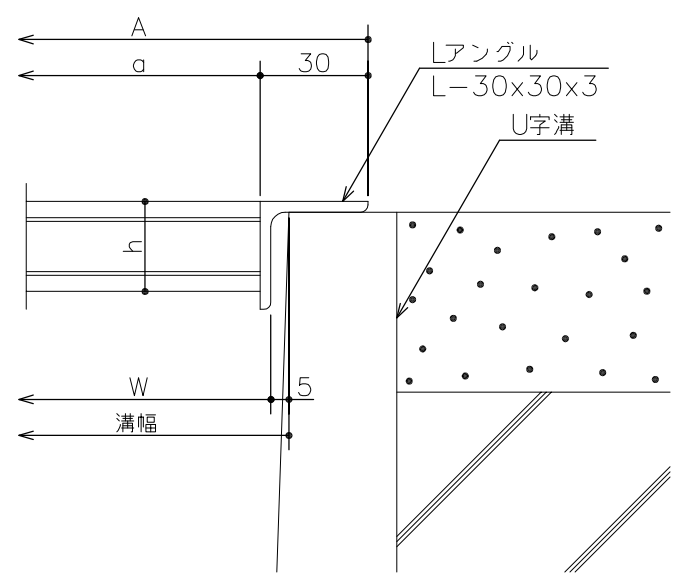
断面詳細図 S=1/2
