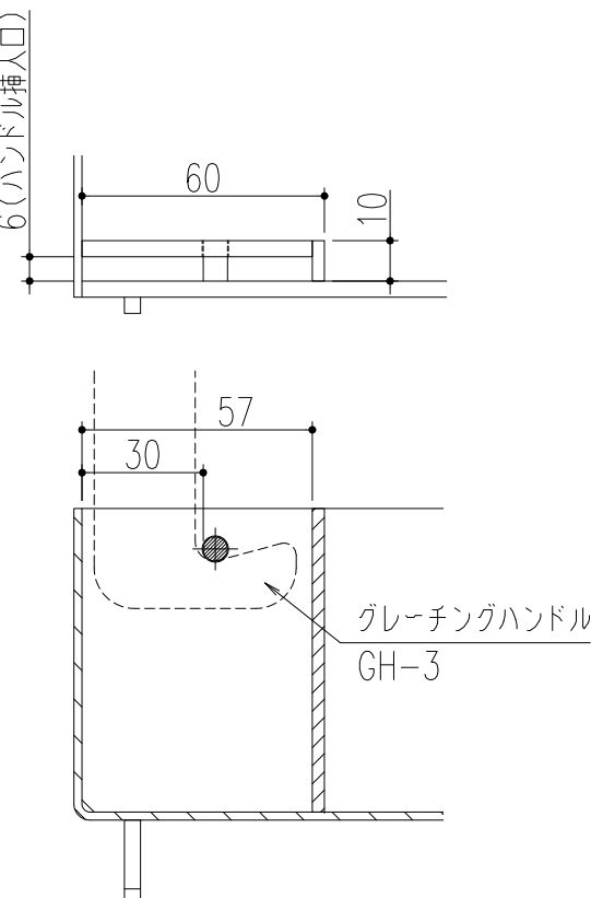
取手部詳細図 (S=1/2)
