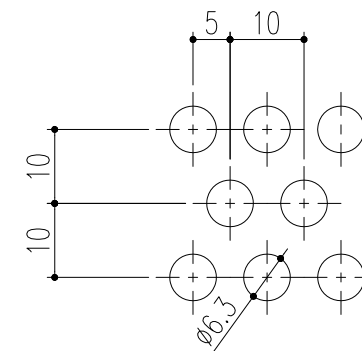
底板 排水穴形状 S=1/1
