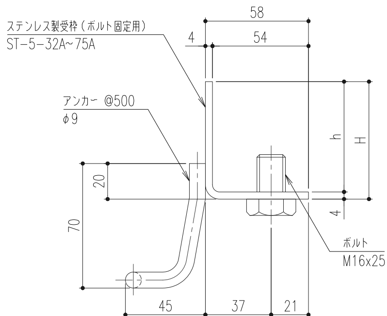
断面詳細図 S=1/2
