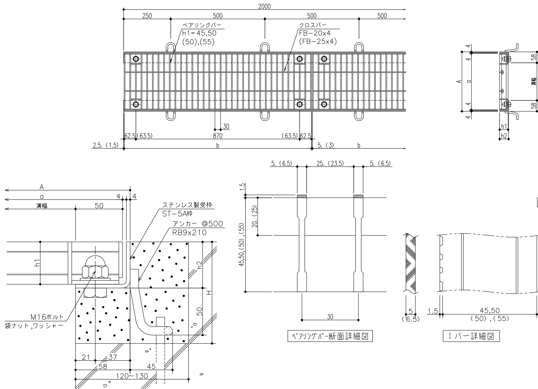
断面詳細図 S=1/2
