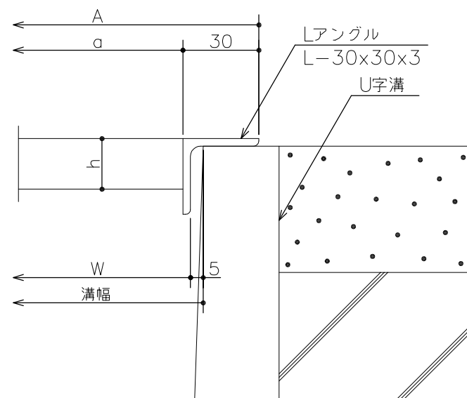
断面詳細図 S=1/2
