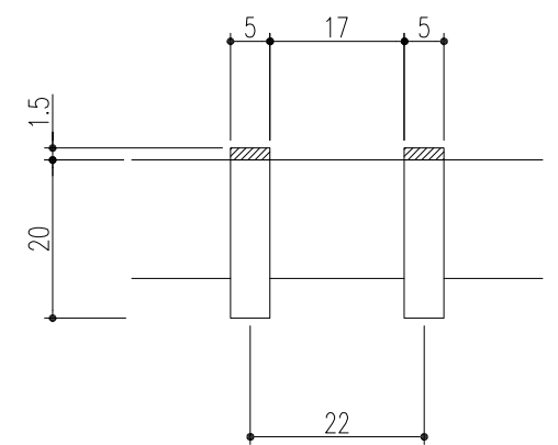
ベアリングバー断面詳細図
