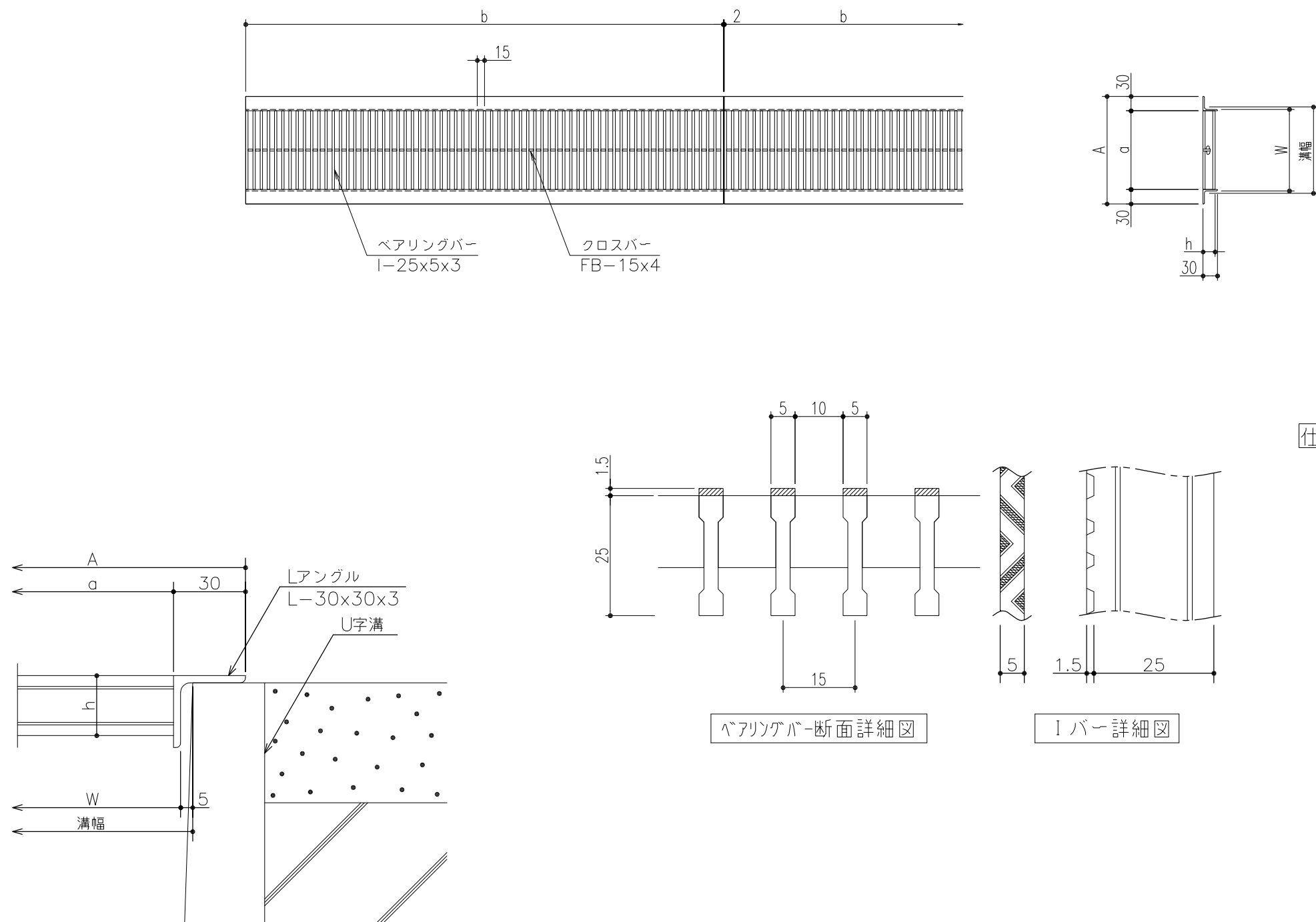
断面詳細図 S=1/2
