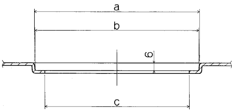
流しトラップ取付け寸法図
