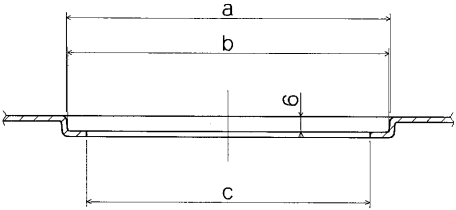
流レトラップ取付け寸法図
