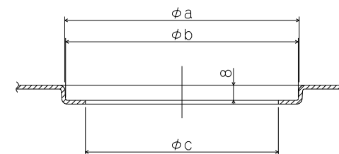
流しトラップ取付け寸法図
