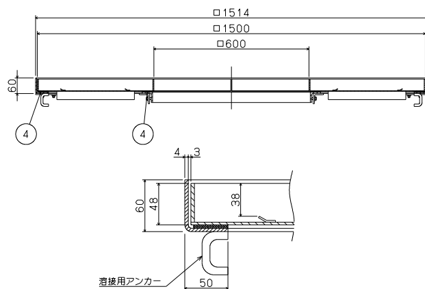
蓋枠嵌合部拡大図
