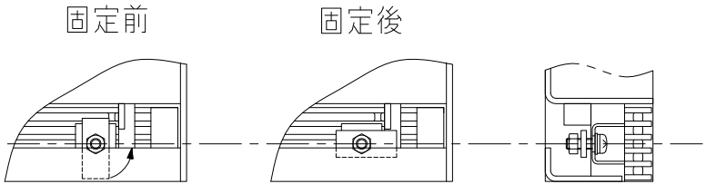
グレーチング固定部詳細図
