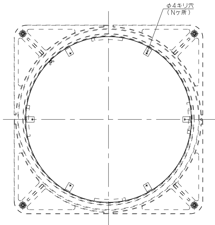
平面図
