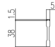
ベアリングバー 詳細図
