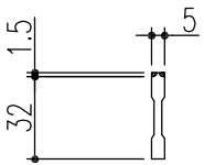
ベアリングバー 詳細図
