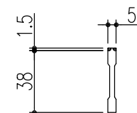
ベアリングバー 詳細図
