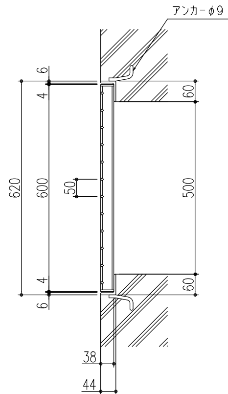
ベアリングバー 詳細図
